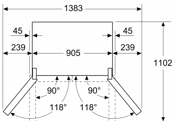
Méretek mm-ben
