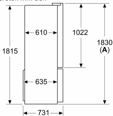
Méretek mm-ben
