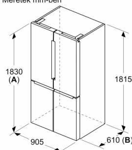
Méretek mm-ben
