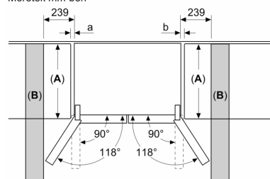
Méretek mm-ben
