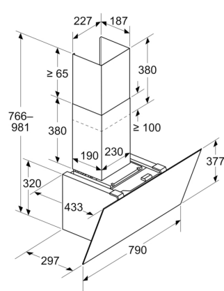
Méretek mm-ben Készülék légkivezetéses üzemmódban
