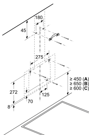
Méretek mm-ben Falra történő szerelés kürtővel
