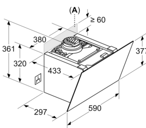
Méretetek mm-ben Készülék levegőkeringetési üzemmódban csatorna nélkül
