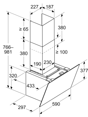
Méretetek mm-ben Készülék légkivezetéses üzemmódban
