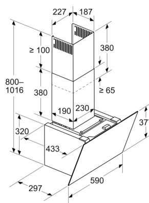
Méretetek mm-ben Készülék levegőkeringetési üzemmódban
