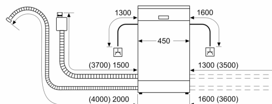
méretetek mm-ben
