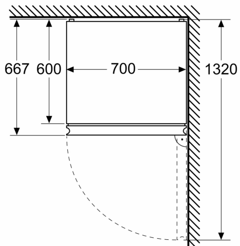
Méretek mm-ben
