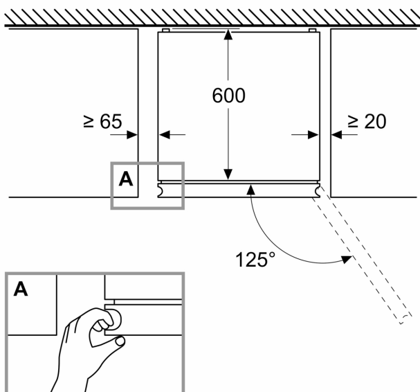
Méretek mm-ben
