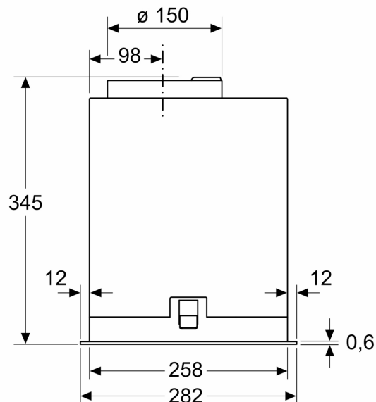
Méretetek mm-ben
