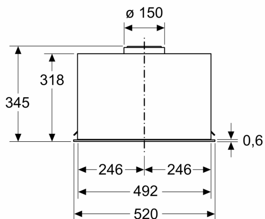
Méretetek mm-ben
