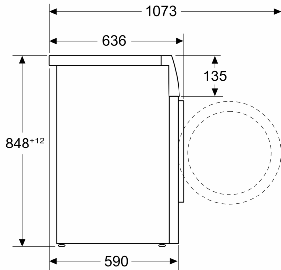
Méreték mm-ben
