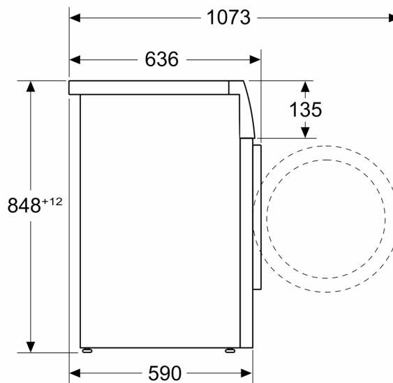
Méreték mm-ben
